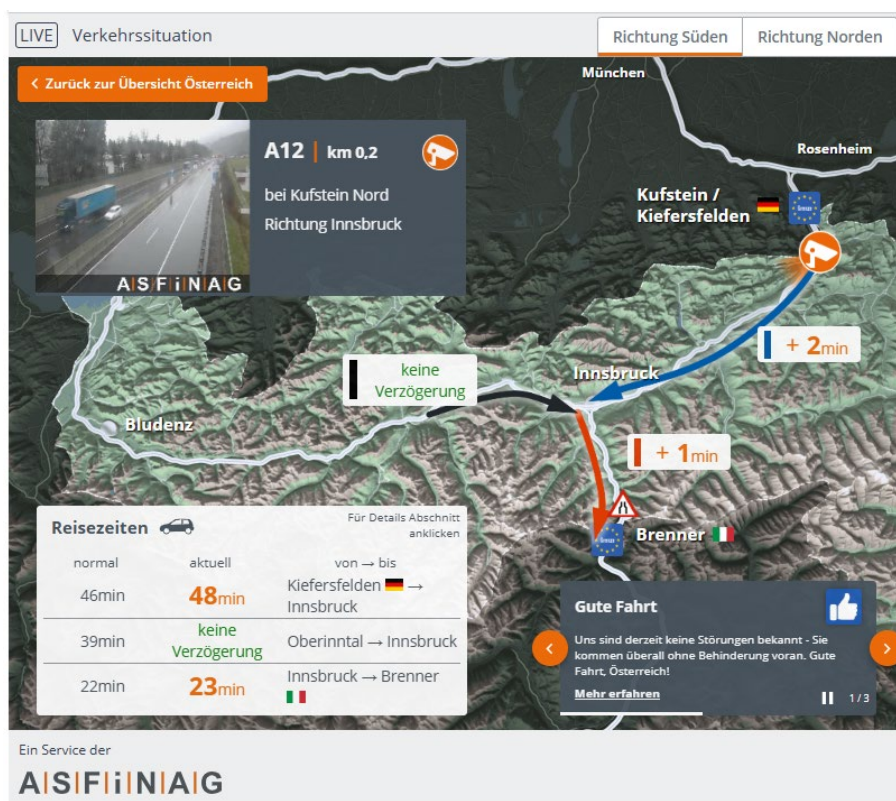
Abbildung 1: Korridor-Widget
